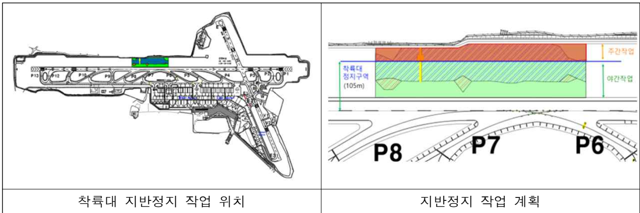
【그림1】 공사 시행 위치도 및 지반정지 작업 계획
