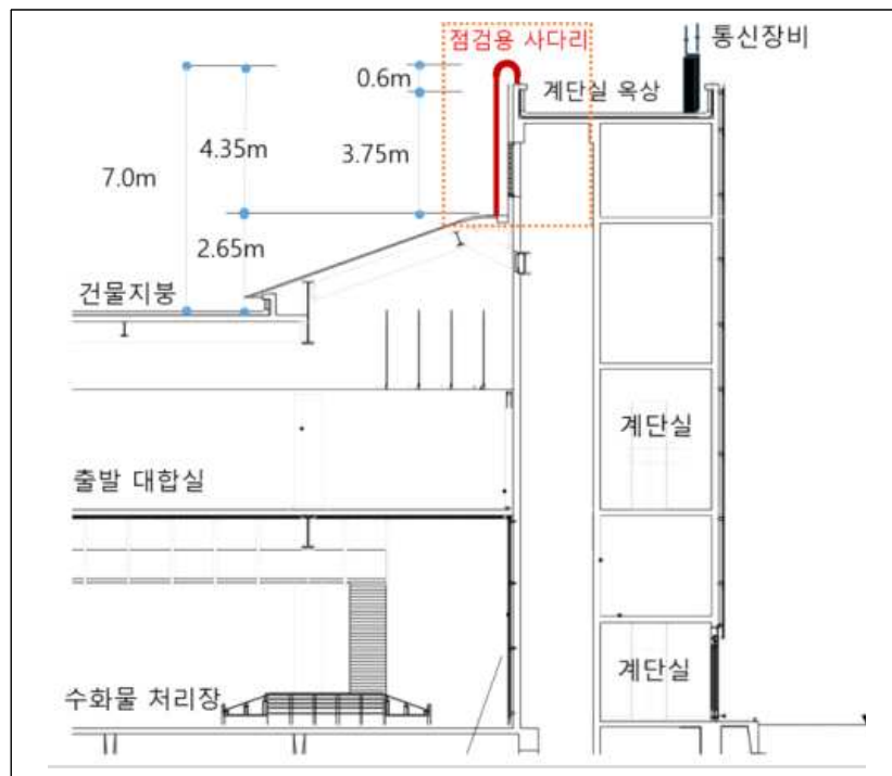
【그림2】 여객청사 단면도 (계단실 옥상 점검용 사다리식 통로)
